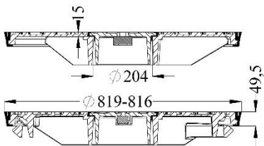
FURNES 3026HT_6503HT
