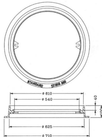
FAST KARM MED PAKNING TYPE STANDARD H = 100 MM
